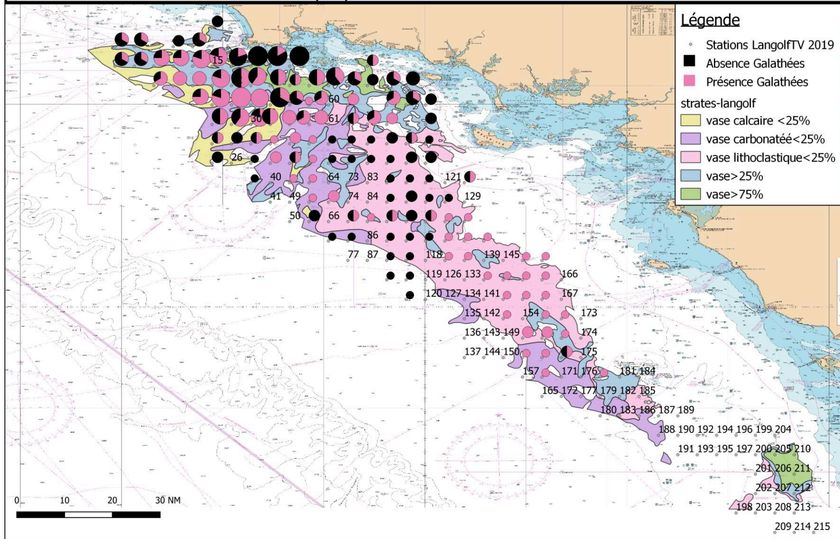
Figure 3 : Réponses concernant la présence de galathées par stations Langolf-TV en fonction du substrat.
