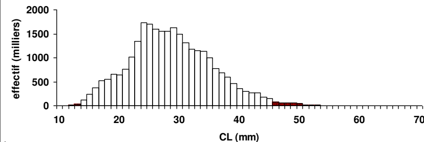
strate lithoclastique (LI)
